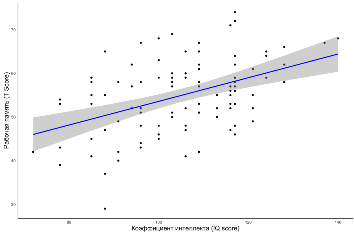
Рисунок 6 — Визуализация корреляции Пирсона между переменной рабочей памяти («Isce Cream») и коэффициентом флюидного интеллекта (CFIT Scale 2, Form A). Каждая точка означает одного участника (N=114)
